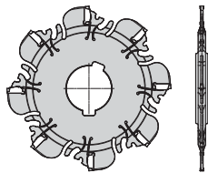
Ausführung für Fräsdornmontage, verstärkter Fräserkörper.
